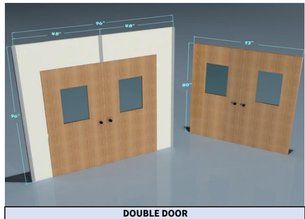
DOUBLE DOOR
