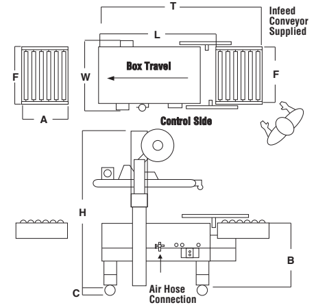
700r & 700rf Footprint
