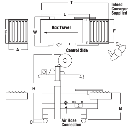
700r & 700r3 Footprint
